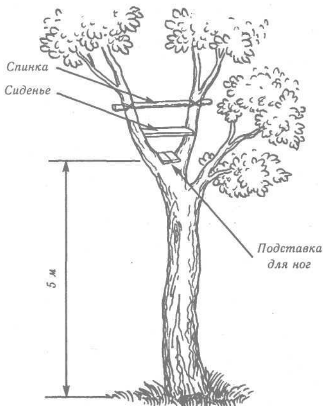
Рис. 2а. Лабаз на одном дереве
